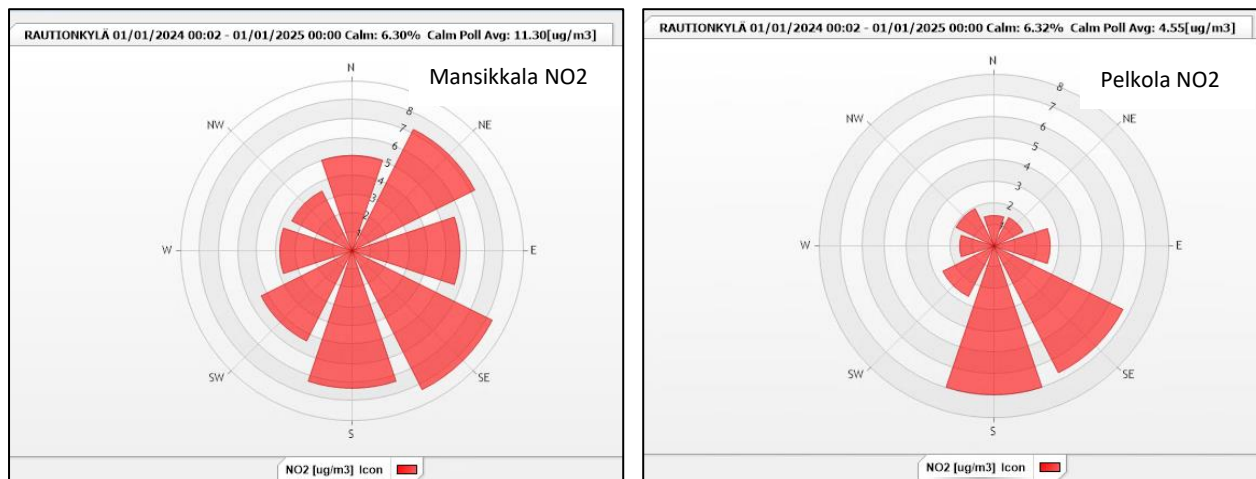
Kuva 22: Imatran Mansikkalan ja Pelkolan mittauspisteiden typidioksidipitoisuuksien ( \mu\text{g}/\text{m}^3 ) tuulensuuntajakaumat vuonna 2024. Rautionkylän tuulensuunta, tuulennopeus \geq 0,3 \text{ m/s} .
