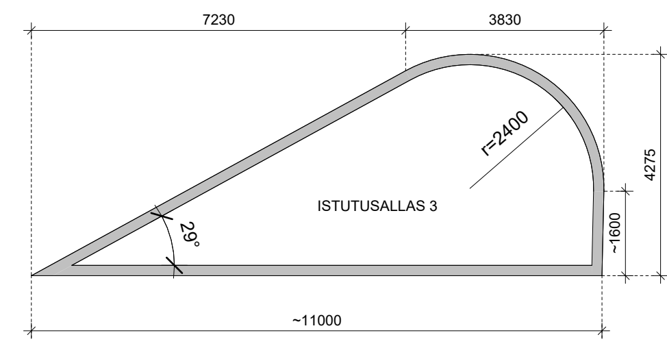
POHJA 1/50 (ISTUTUSALLAS 3)
