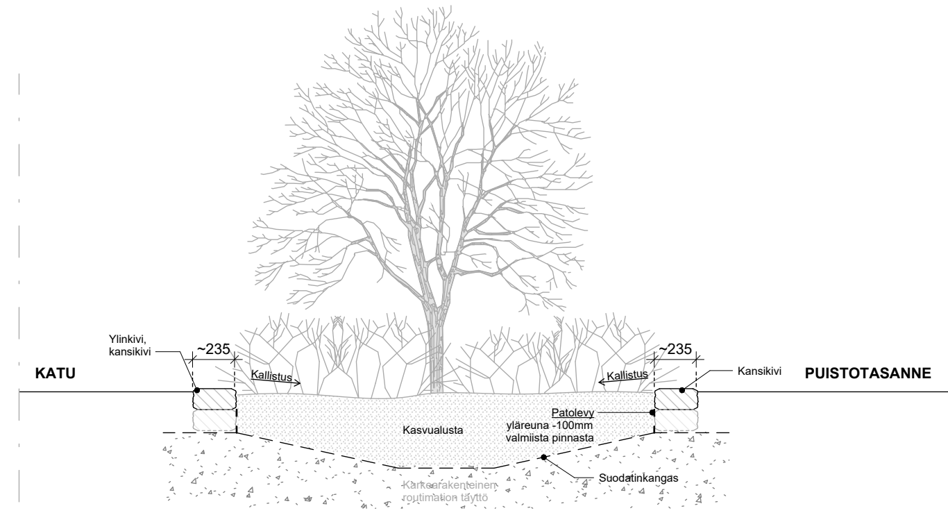
LEIKKAUS I3 1/25 (ISTUTUSALLAS 3)
