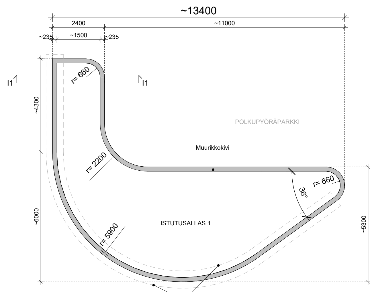
POHJA 1/50 (ISTUTUSALLAS 1)
