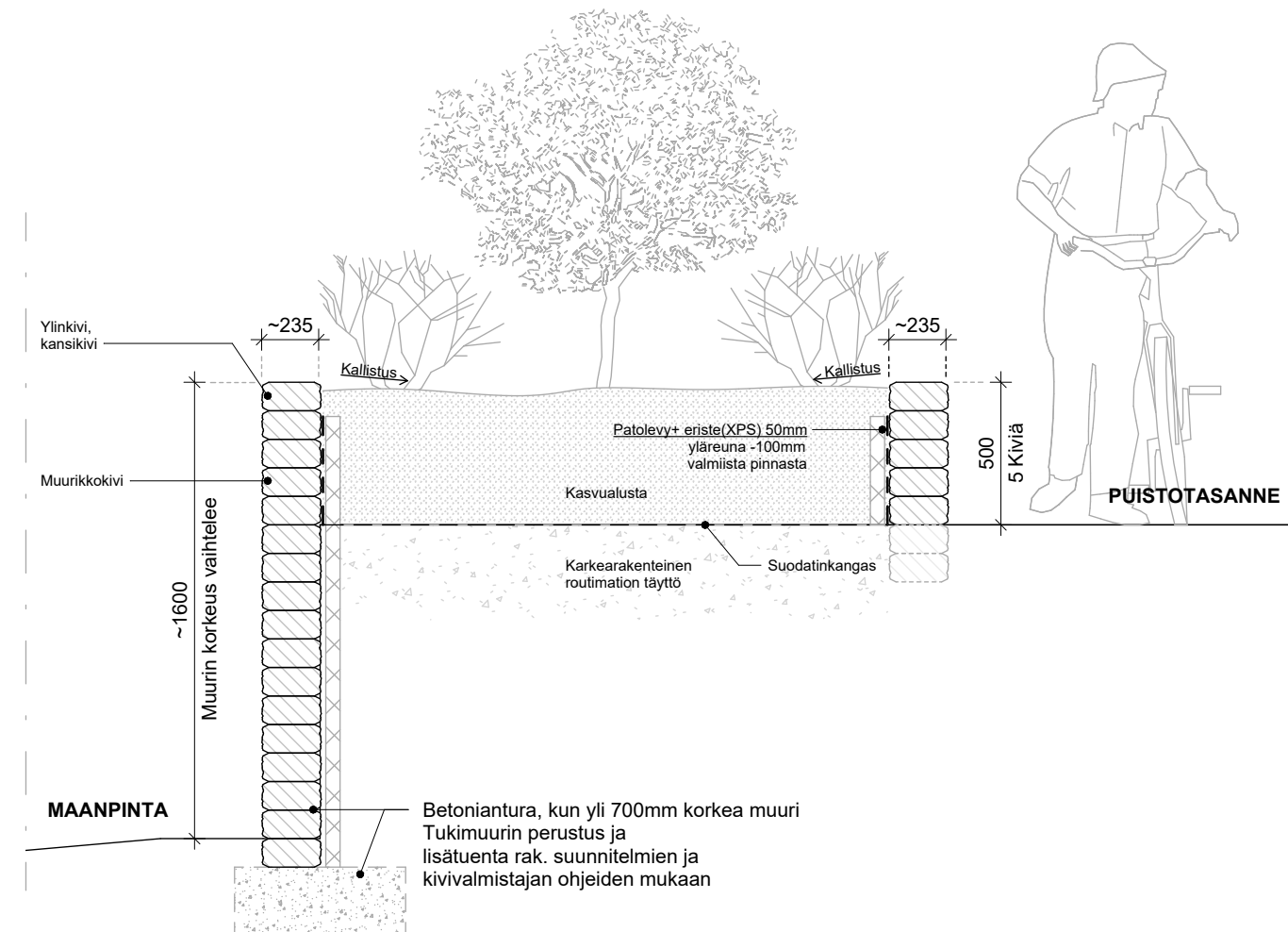
LEIKKAUS I1 1/25 (ISTUTUSALLAS 1)
