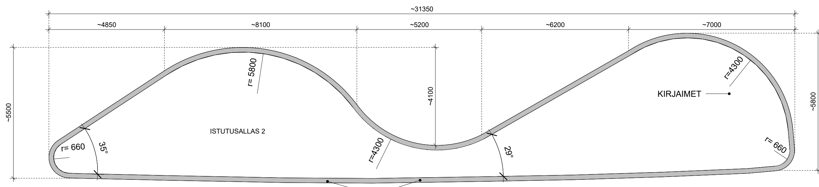
POHJA 1/50 (ISTUTUSALLAS 2)
