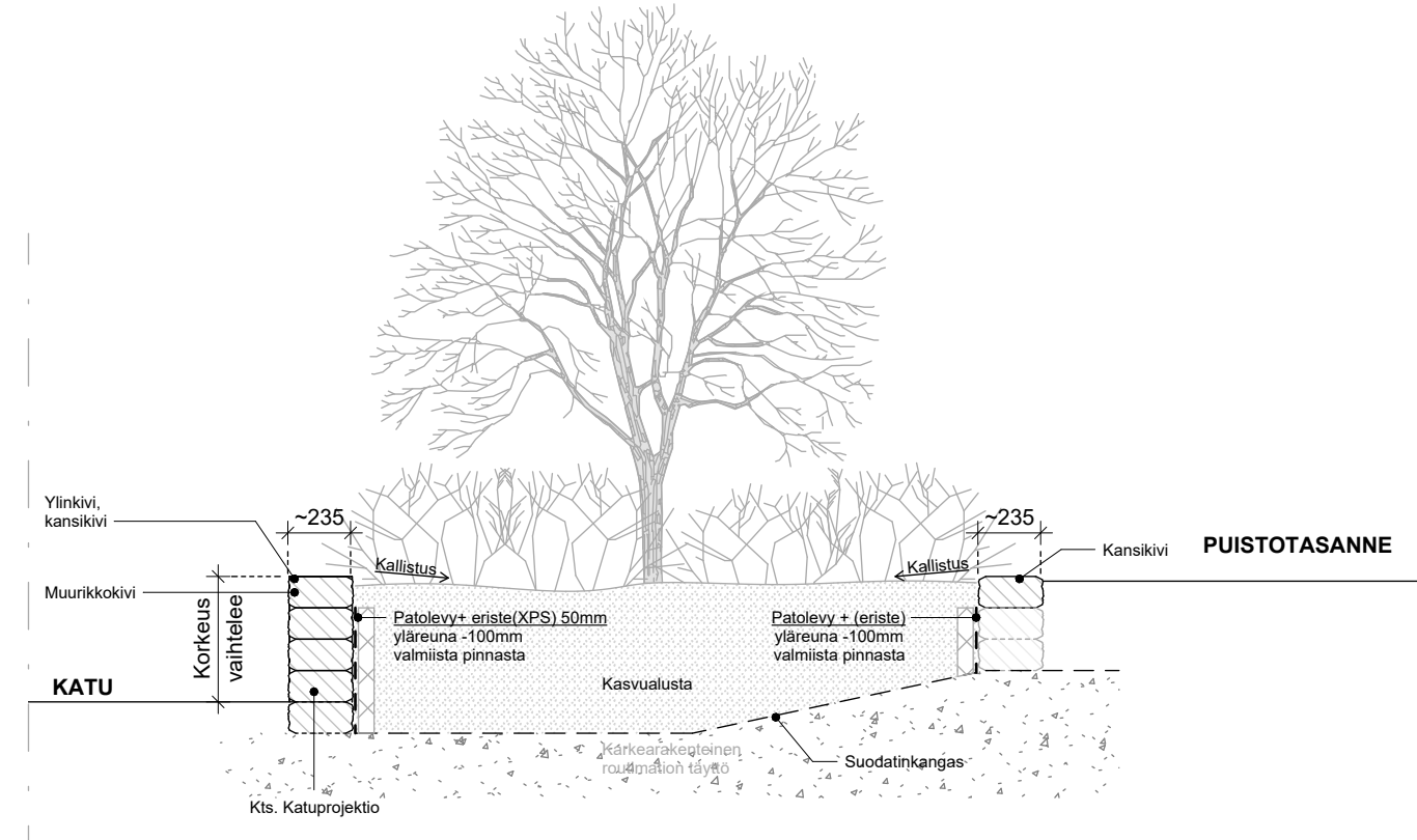
LEIKKAUS I2 1/25 (ISTUTUSALLAS 2)
